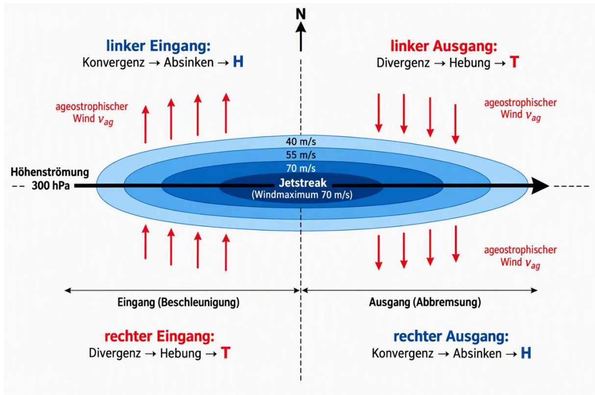
Abbildung 10: Vier-Quadranten-Modell eines Jetstreaks (Nordhalbkugel) – ageostrophische Windvektoren, Divergenz im rechten Eingang und linken Ausgang (Tiefentwicklung), Konvergenz im linken Eingang und rechten Ausgang
