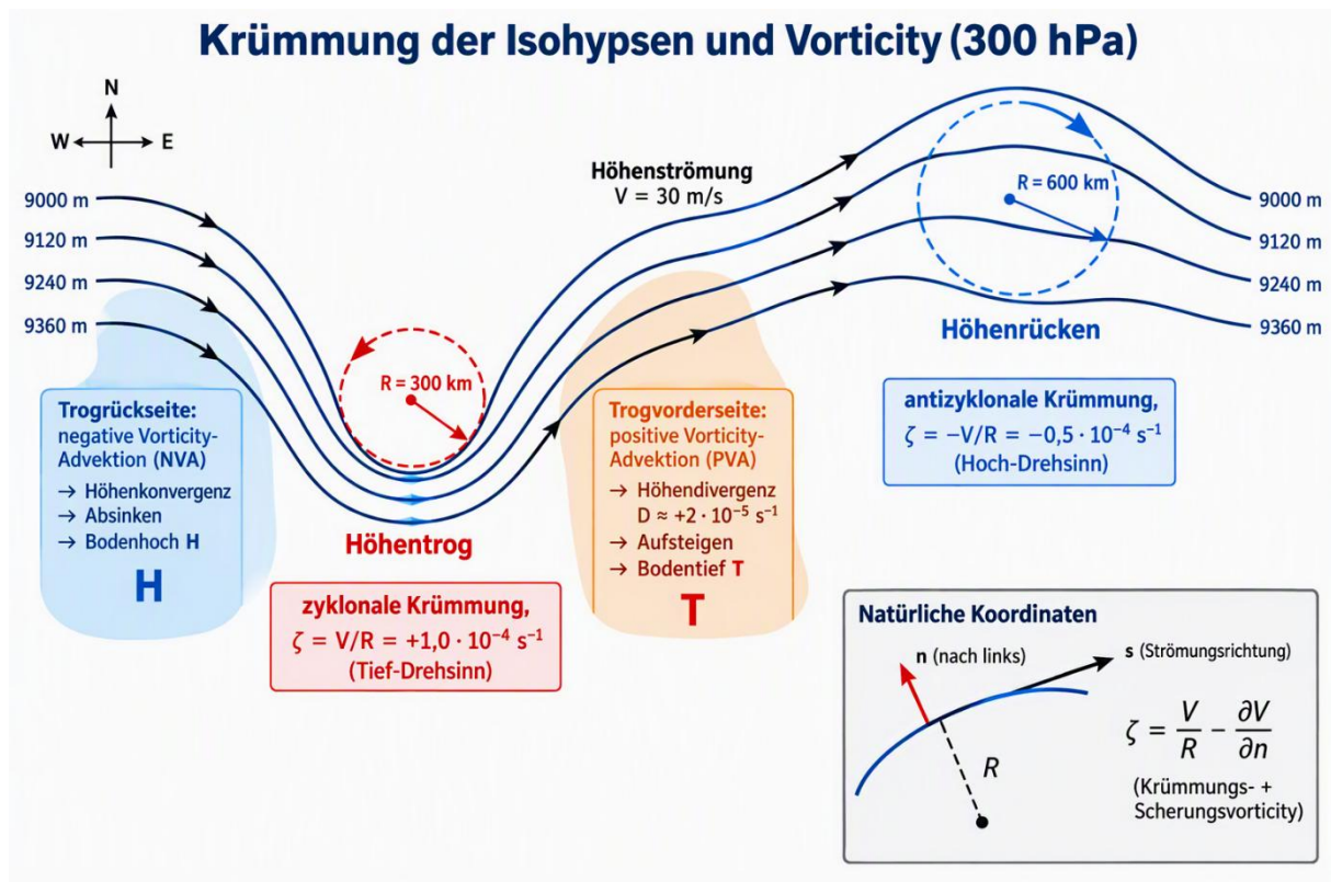
Abbildung 11: Krümmung der Isohypsen und Vorticity (300 hPa) – zyklonale Krümmung im Höhentrog ( R = 300 \text{ km} , \zeta = +1,0 \times 10^{-4} \text{ s}^{-1} ), antizyklonale Krümmung im Höhenrücken ( R = 600 \text{ km} , \zeta = -0,5 \times 10^{-4} \text{ s}^{-1} ); auf der Trogvorderseite positive Vorticity-Advektion mit Höhendivergenz und Bodentief, auf der Trogrückseite negative Vorticity-Advektion mit Konvergenz und Bodenhoch (Werte aus Beispiel 17)
