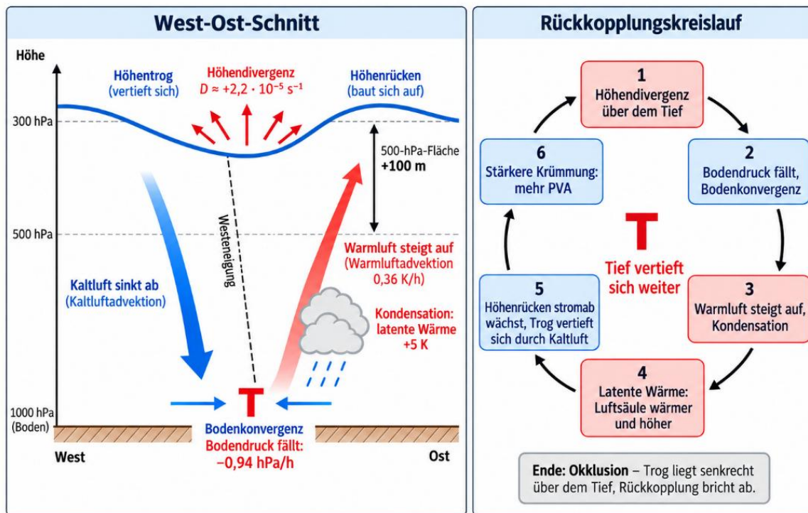
Abbildung 12: Selbstverstärkung eines Tiefs – links West-Ost-Schnitt mit aufsteigender Warmluft und Freisetzung latenter Wärme (+5 K, 500-hPa-Fläche +100 m), absinkender Kaltluft, Westneigung und Höhendivergenz über dem Bodentief (Druckfall -0,94 \text{ hPa/h} ); rechts Rückkopplungskreislauf bis zur Okklusion (Werte aus den Beispielen 12, 17, 18 und 19)
