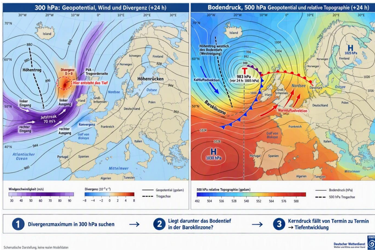
Abbildung 14: Idealisierte Vorhersagekarte einer Tiefentwicklung (+24 h) – links 300 hPa mit Jetstreak (70 m/s) und Höhendivergenz im linken Ausgang, rechts Bodendruck, 500-hPa-Geopotential und relative Topografie mit Baroklinzone und Westneigung des Höhentrogs; Kerndruck von 1005 auf 983 hPa in 24 h (Werte aus den Beispielen 16, 17 und 19). Schematische Darstellung, keine realen Modelldaten
