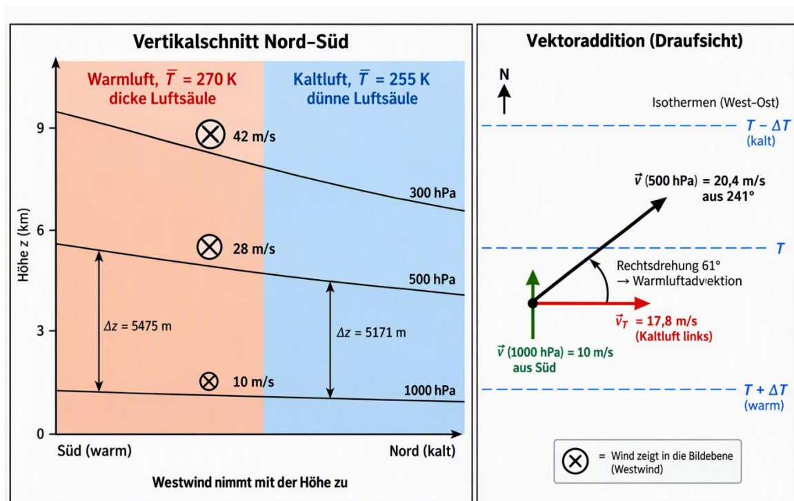
Abbildung 7: Thermischer Wind – links Nord-Süd-Schnitt mit Schichtdicken (1000–500 hPa), nach Norden geneigten Druckflächen und mit der Höhe zunehmendem Westwind; rechts Vektoraddition \vec{v}(500\text{ hPa}) = \vec{v}(1000\text{ hPa}) + \vec{v}_T mit Rechtsdrehung (Warmluftadvektion)
