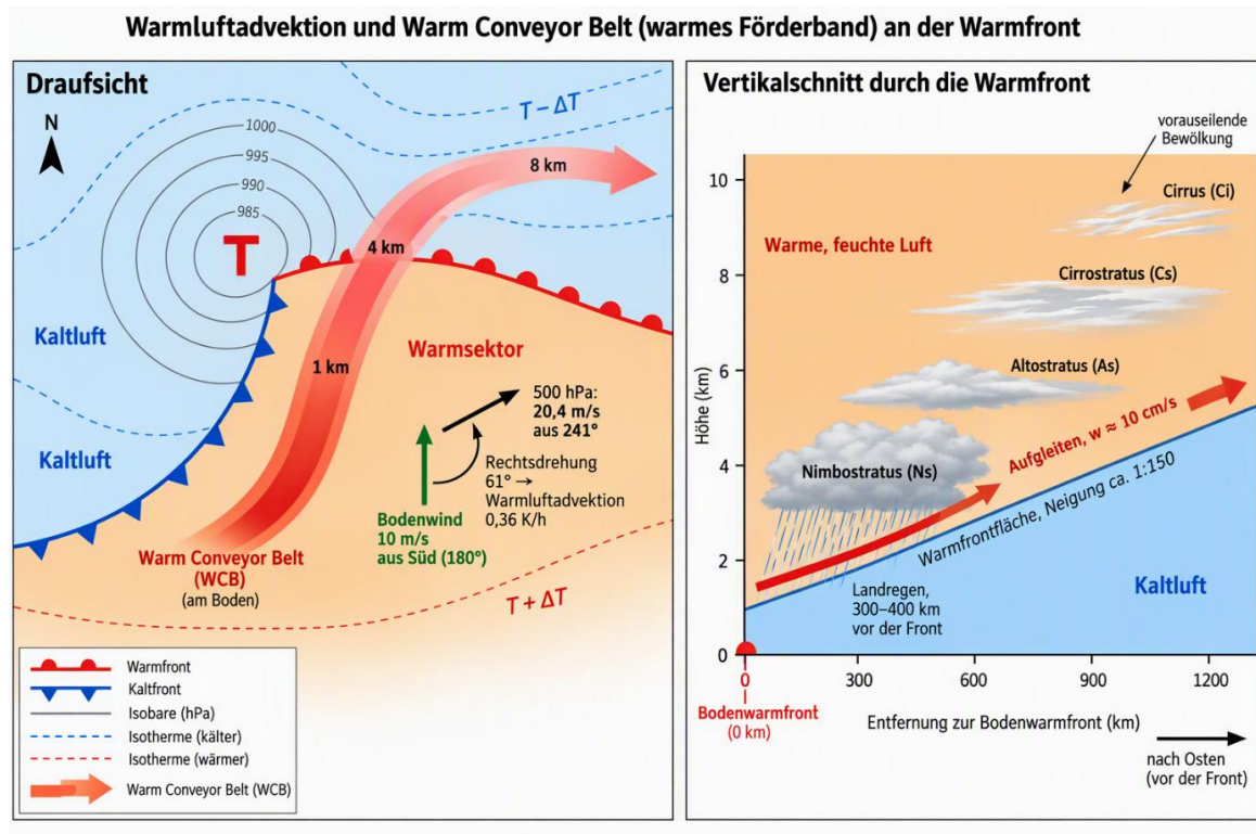
Abbildung 8: Warmluftadvektion und Warm Conveyor Belt – links Draufsicht mit Warmsektor, Fronten, Förderband und Rechtsdrehung des Windes mit der Höhe (Werte aus Beispiel 12); rechts Vertikalschnitt durch die Warmfront mit Aufgleiten (Neigung ca. 1:150) und vorausseilender Bewölkung (Ci, Cs, As, Ns)
