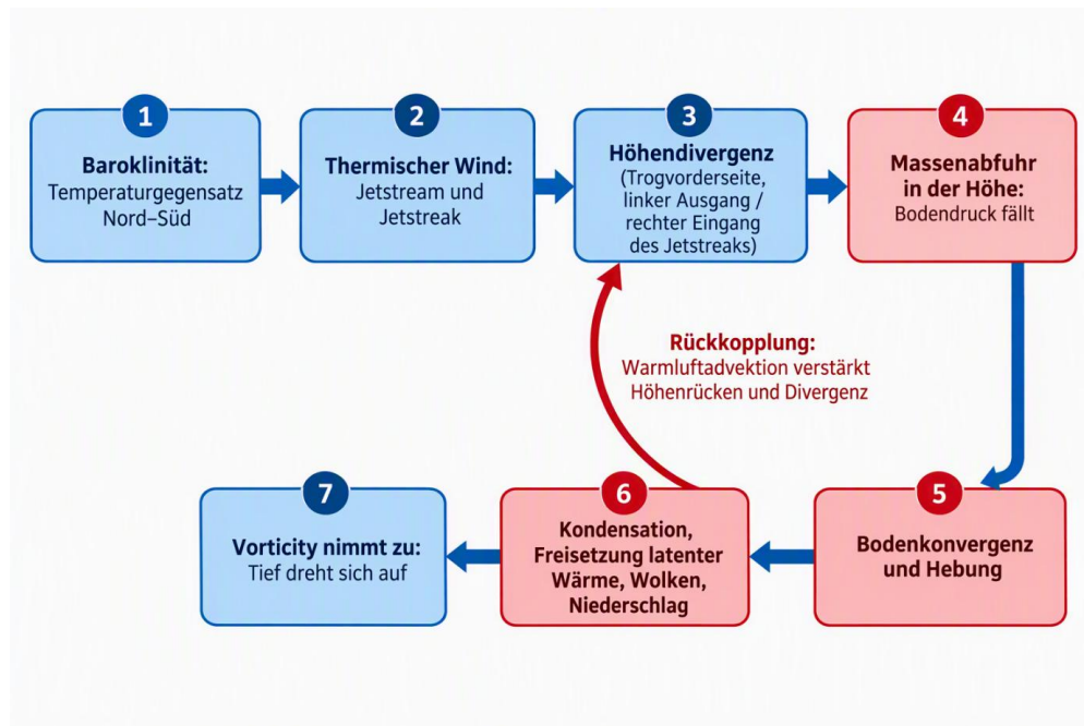
Abbildung 13: Wirkungskette der dynamischen Tiefdruckentwicklung mit Rückkopplung
