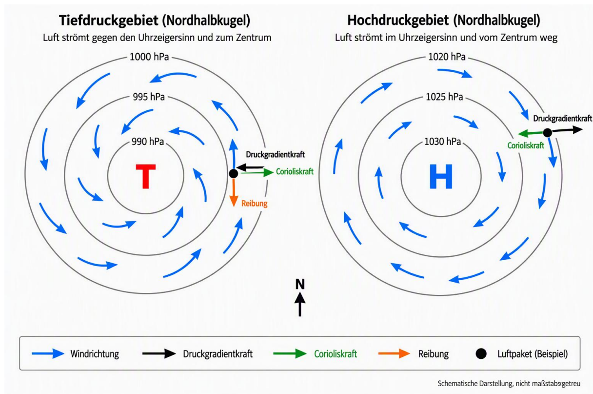
Abbildung 2: Kräftevektoren (Druckgradientkraft, Corioliskraft, Reibung) und bodennahes Windfeld um ein Tief (links) und ein Hoch (rechts) auf der Nordhalbkugel
