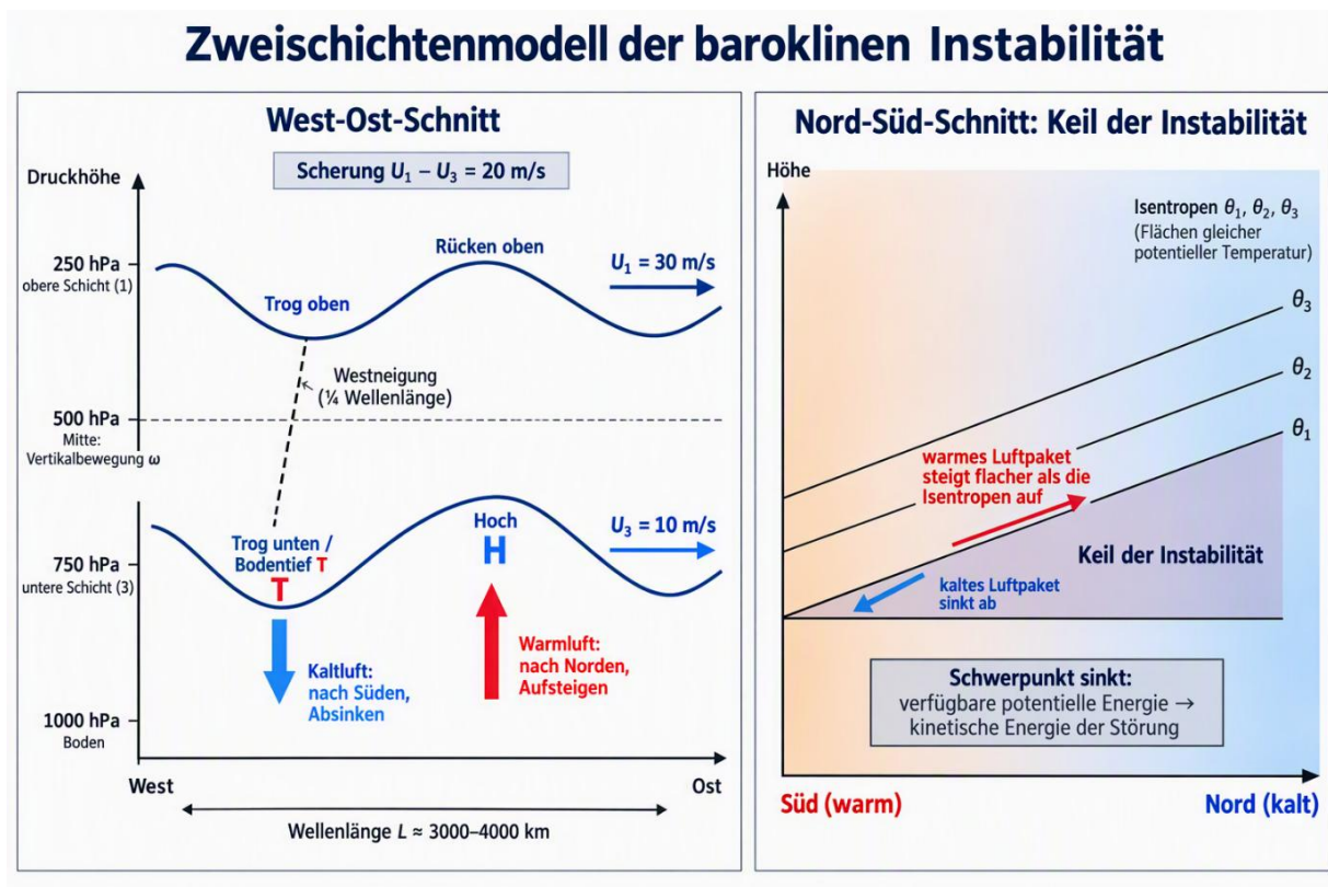
Abbildung 9: Zweischichtenmodell der baroklinen Instabilität – links West-Ost-Schnitt mit oberer(250 hPa) und unterer Schicht (750 hPa), Westneigung der Welle, Aufsteigen der Warmluft
