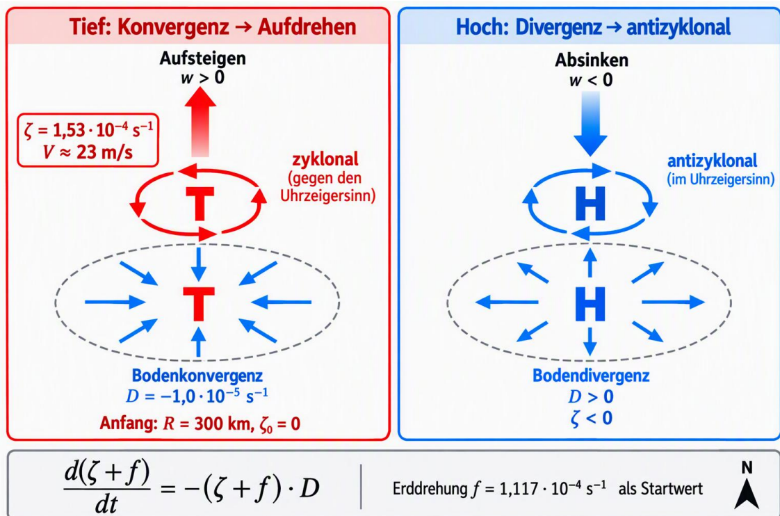
Abbildung 5: Vorticity – Bodenkonvergenz zieht die Luftsäule zusammen und lässt sie zyklonal aufdrehen (Tief, links); Bodendivergenz erzeugt antizyklonale Drehung (Hoch, rechts). Werte aus Beispiel 7
