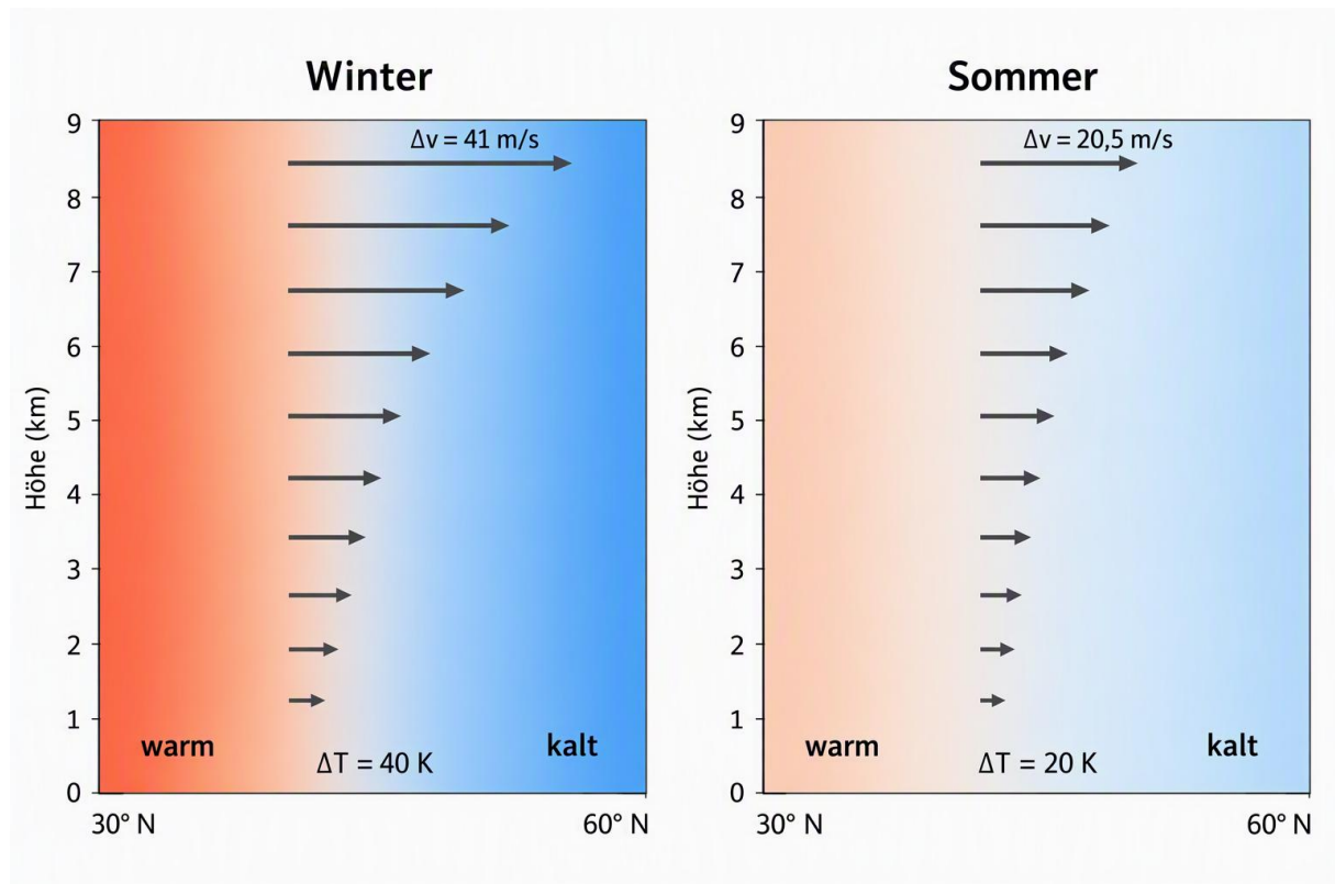
Abbildung 7a: Jetstream im Winter und im Sommer – Nord-Süd-Schnitt zwischen 30° N und 60° N; der doppelt so große Temperaturgegensatz im Winter ( \Delta T = 40 \text{ K} statt 20 \text{ K} ) verdoppelt die Windzunahme mit der Höhe ( \Delta v_T \approx 41 \text{ m/s} statt 20,5 \text{ m/s} ). Werte aus Beispiel 11
