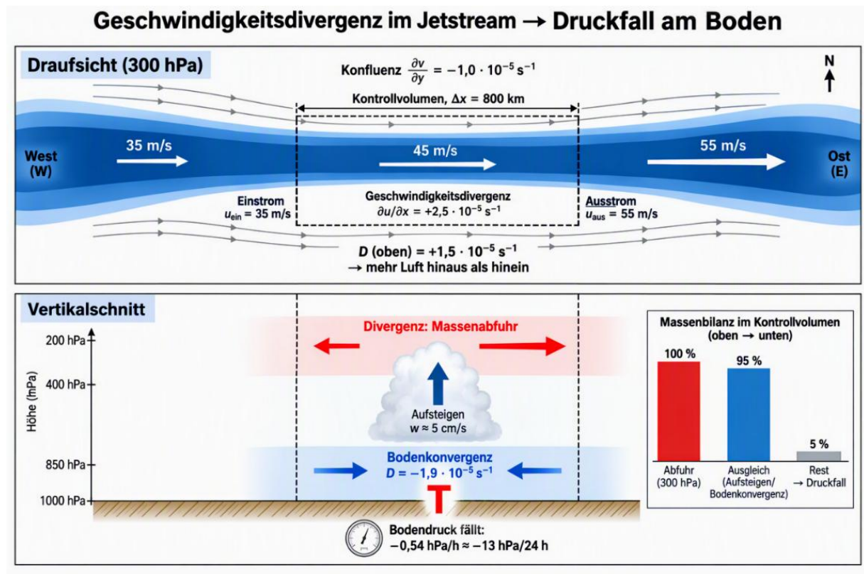
Abbildung 4: Geschwindigkeitsdivergenz im Jetstream – oben Draufsicht: Die Luft wird entlang des Jets von 35 auf 55 m/s beschleunigt, aus dem Kontrollvolumen strömt mehr Luft heraus als hinein; unten Vertikalschnitt: Massenabfuhr in der Höhe, Bodenkonvergenz, Aufsteigen und Druckfall am Boden (Werte aus dem Zahlenbeispiel in Abschnitt 3.2)
