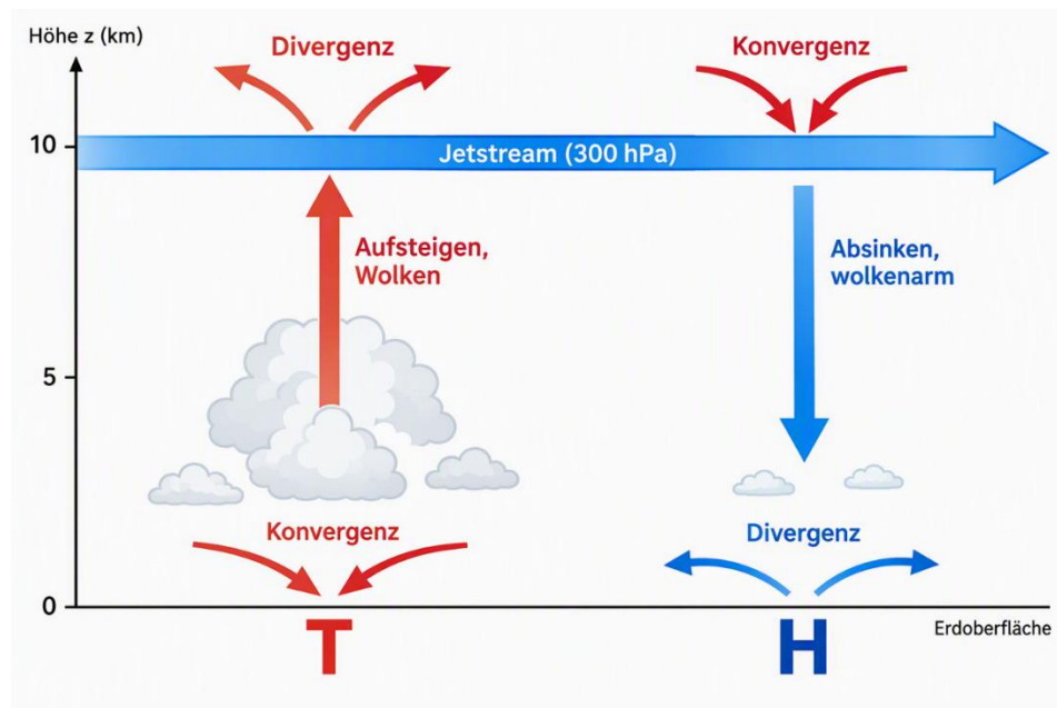
Abbildung 3: Vertikalschnitt – Divergenz am Jetstream über dem Bodentief (Aufsteigen) und Konvergenz in der Höhe über dem Bodenhoch (Absinken)
